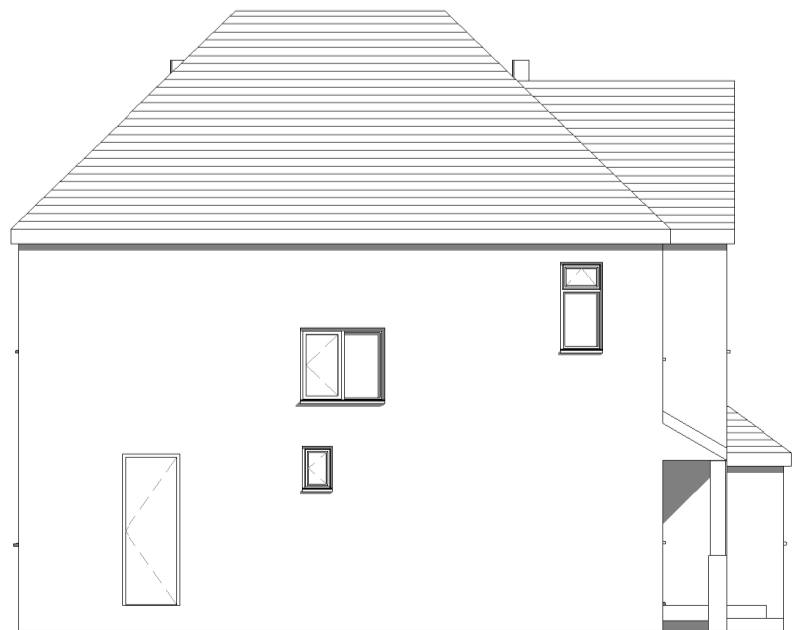
Existing Side R 1 : 100
