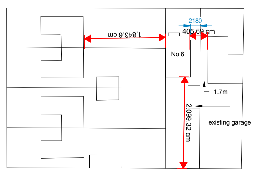
Site Plan Existing1 1 : 500
