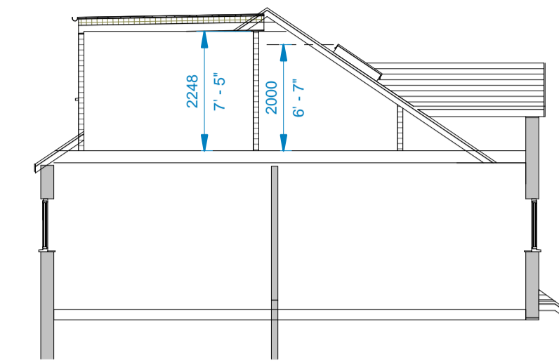
Section 1 1 : 100
